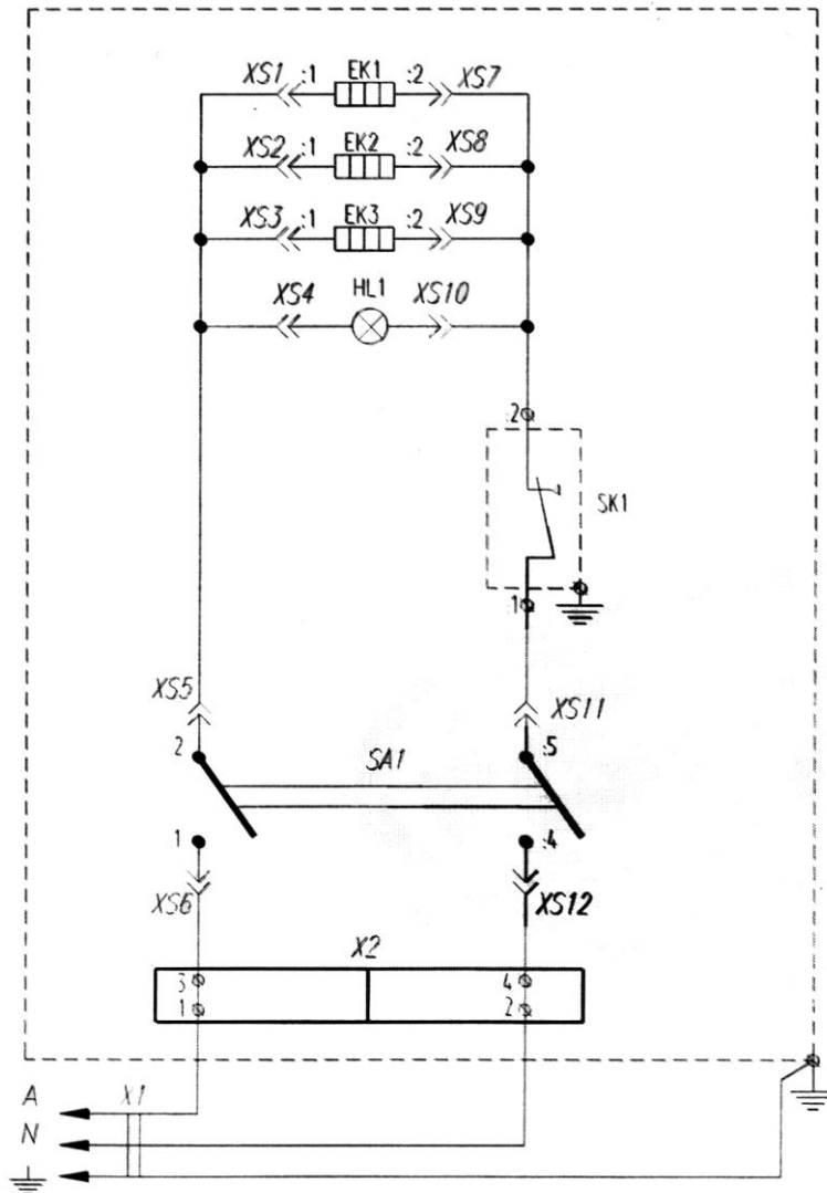
Рисунок 3. Схема электрическая принципиальная.
