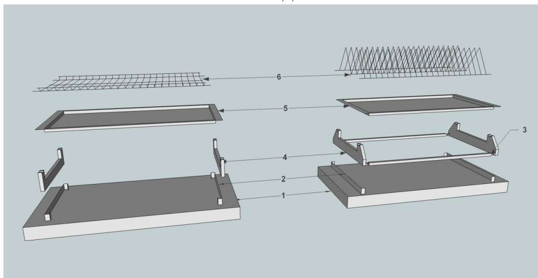
Рис.1 Схема сборки полки ПКс, ПКт, для сушки посуды.(тарелок, стаканов)
